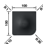
CapFlow – kryt na výpušť není možné kombinovat s InFino®
